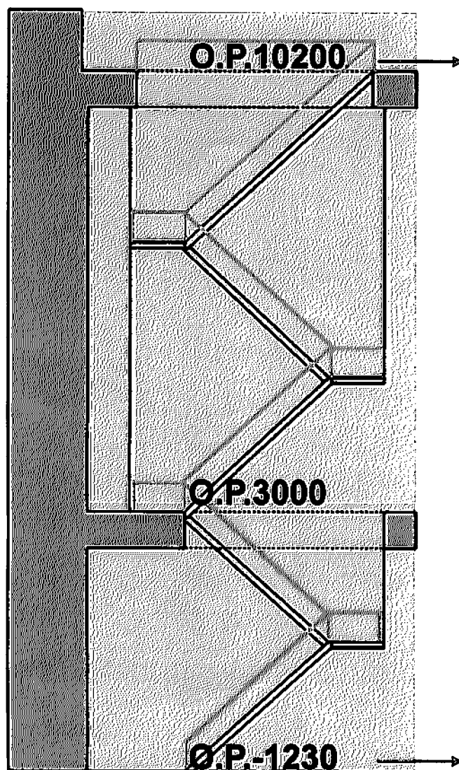
北西階段 断面図
