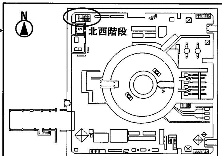
原子炉建屋 地上階 平面図
