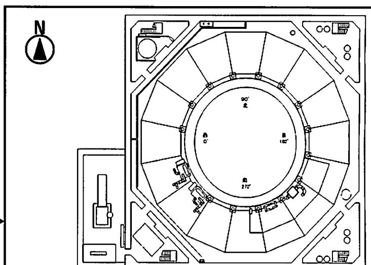
原子炉建屋 地下階 平面図
